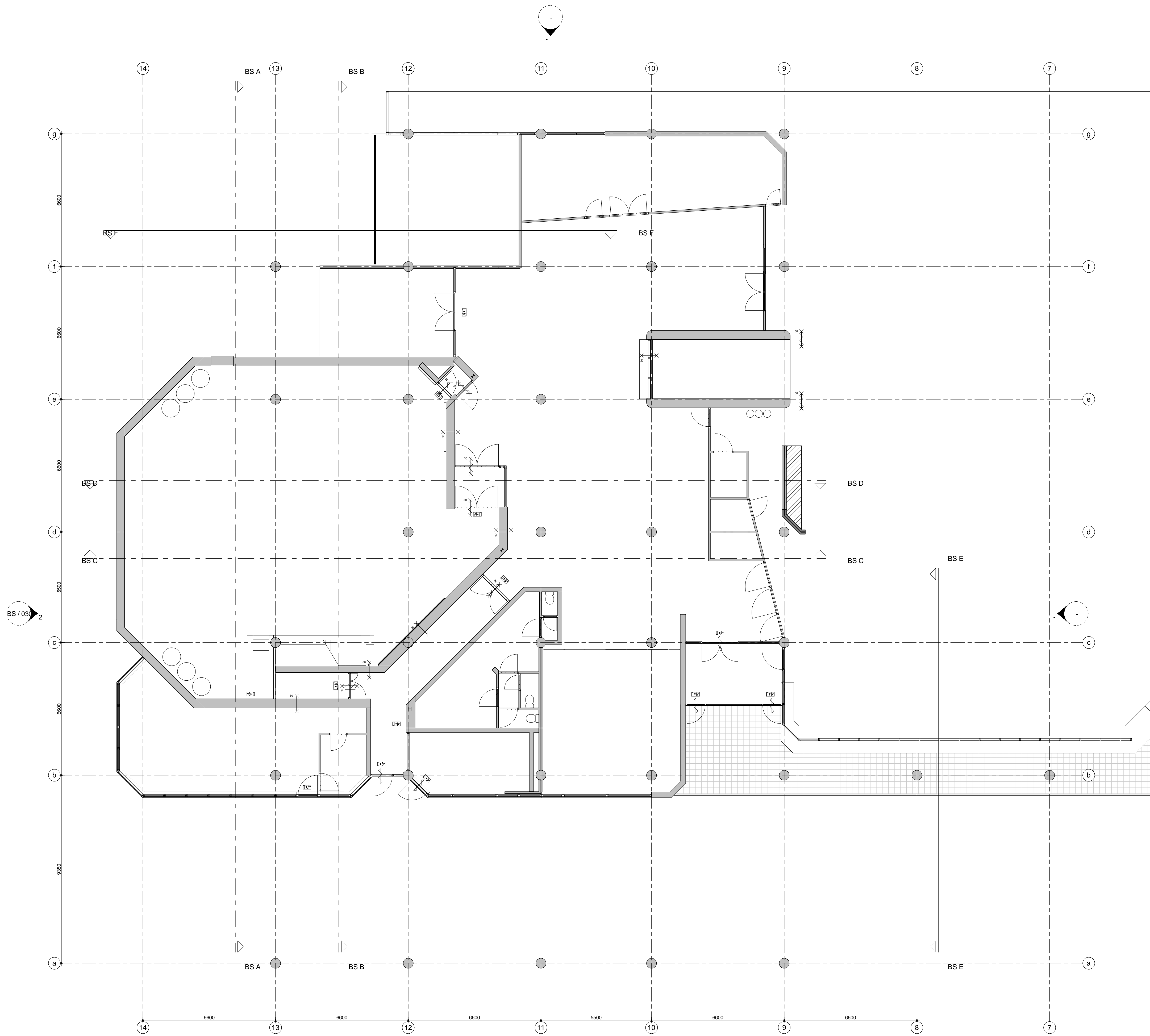
begane grond bestaande situatie
